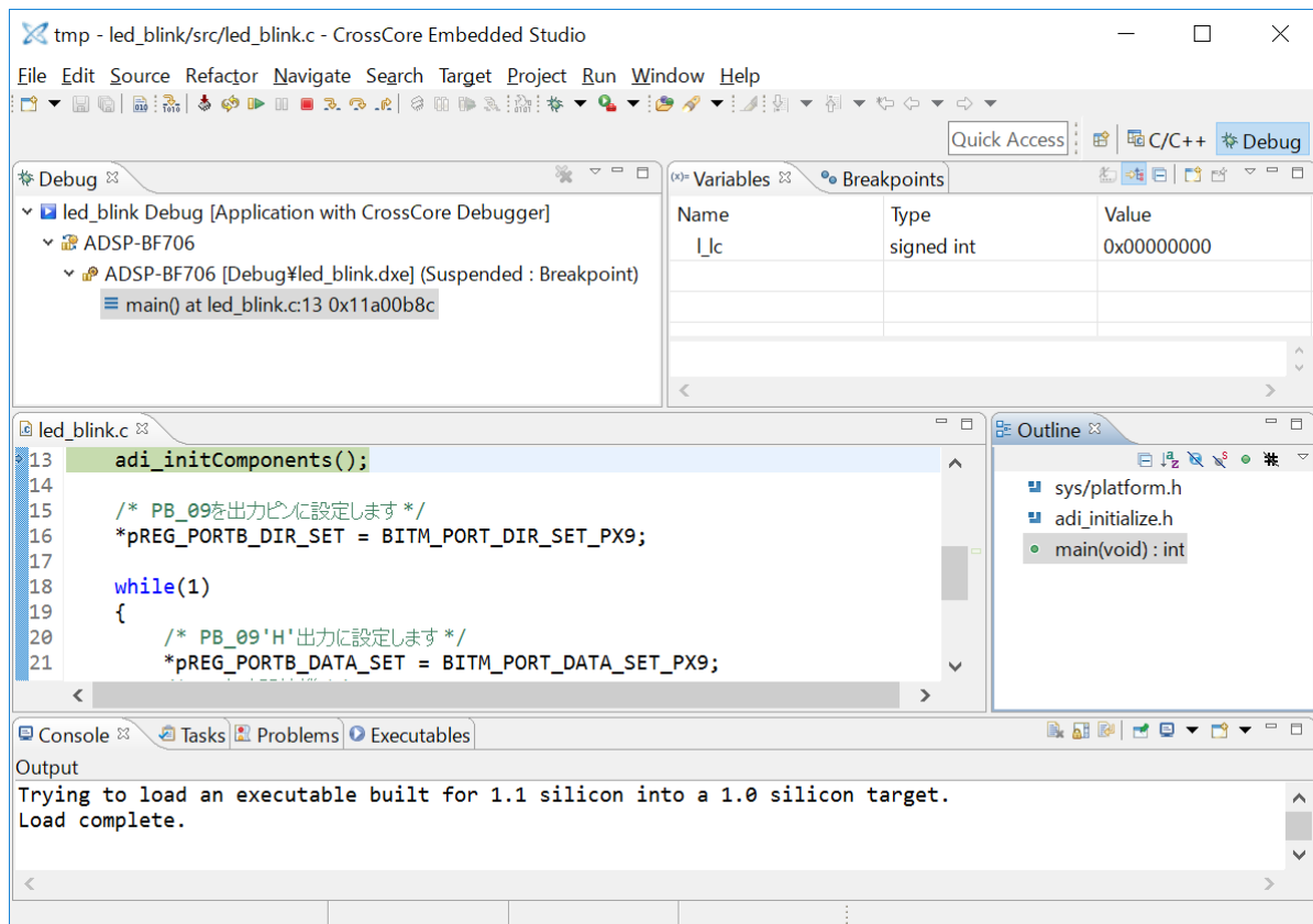
図 38 デバッグ画面
