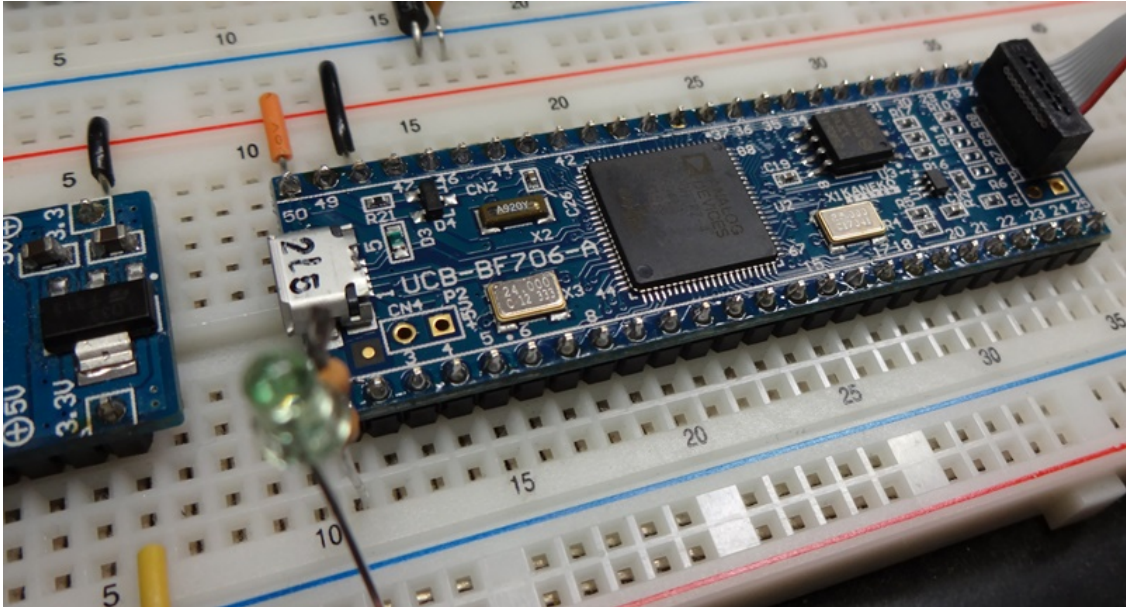
図 29 JTAG-ICE 接続例
