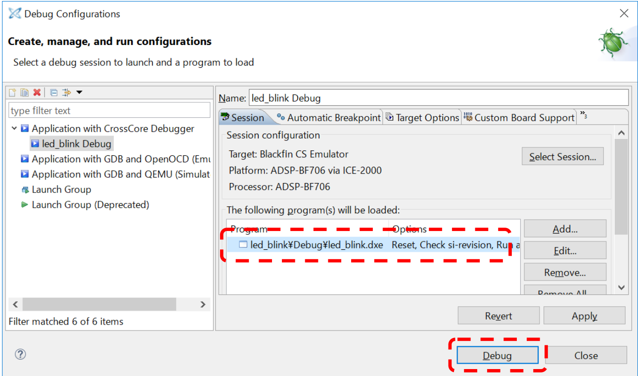
図 35 Debug Configuration 画面
