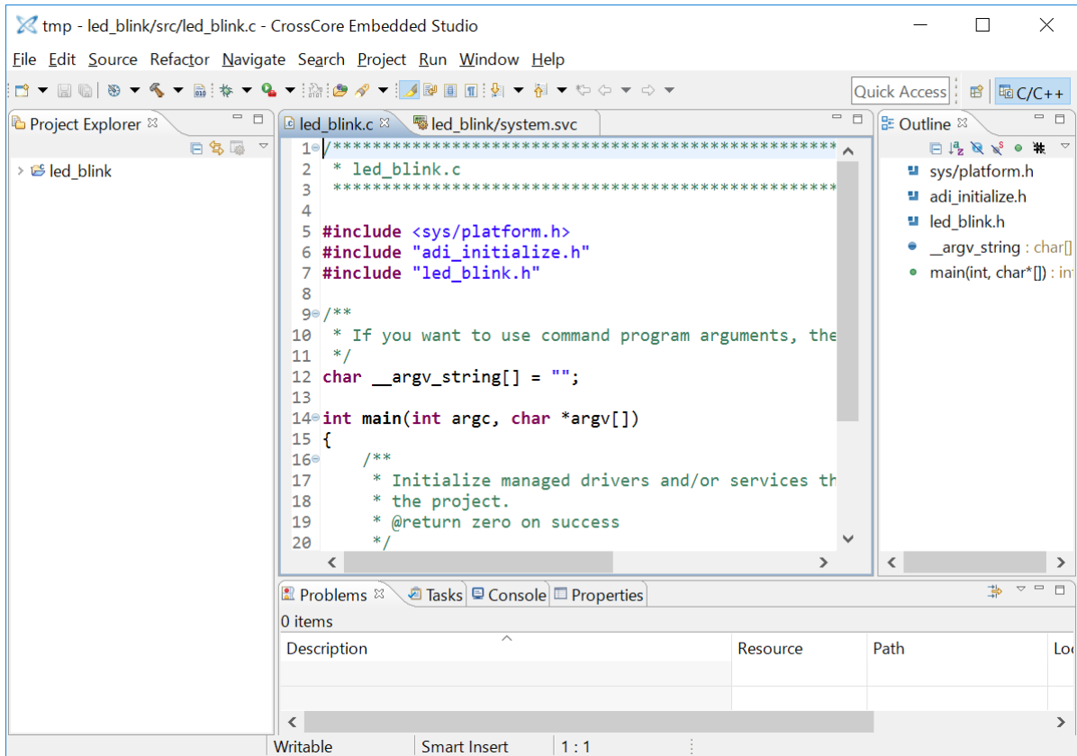
図 27 CrossCore Embedded Studio IDE 画面（プロジェクト追加）
