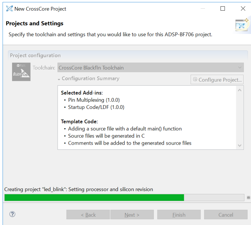
図 26 New CrossCore Project ダイアログ (プロジェクト生成)
