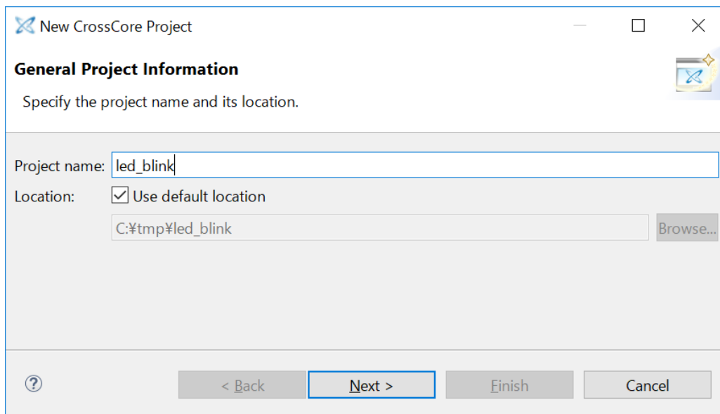
図 23 New CrossCore Project ダイアログ (プロジェクト名指定)
